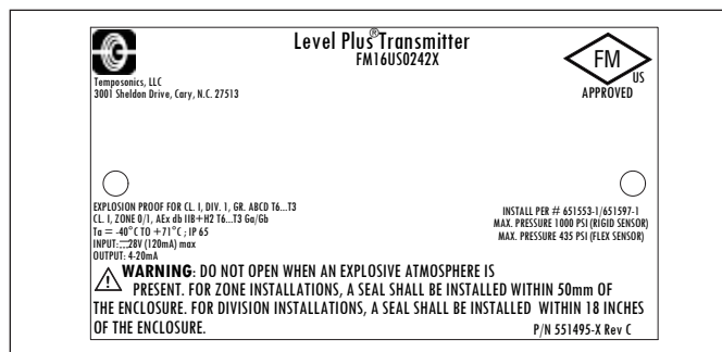
Fig. 26 : Antidéflagrant, étiquette FM, HART®, option de boîtier D, E
