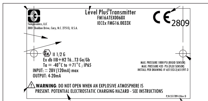
Fig. 60 : Ininflammable, étiquette ATEX et IECEx, HART®, option de boîtier D, E, G, H, ou L
