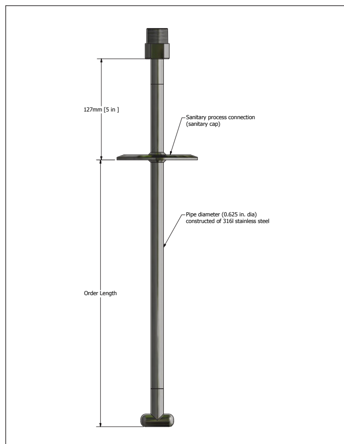
Fig. 5 : Configuration du tube extérieur
