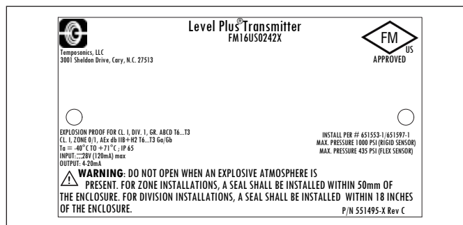
Fig. 25 : Antidéflagrant, étiquette FM, HART®, option de boîtier Option G, H, ou L
