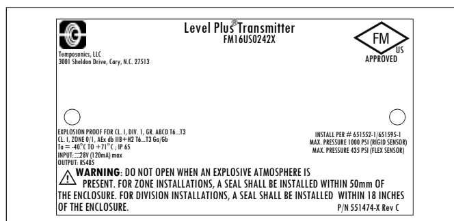
Fig. 24 : Antidéflagrant, étiquette FM, Modbus ou DDA, option de boîtier D, E
