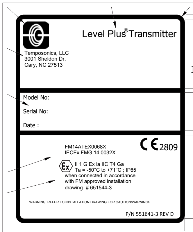
Fig. 52 : Étiquette ATEX/IECEX sécurité intrinsèque, Modbus ou DDA, boîtier NEMA
