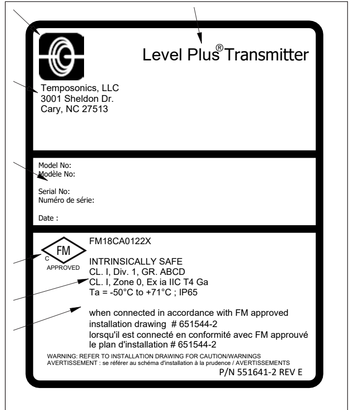
Fig. 32 : Étiquette FMC sécurité intrinsèque, HART®, boîtier NEMA
